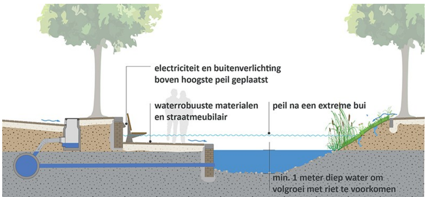
Schematische doorsnede van een stadsuiterwaarde.
